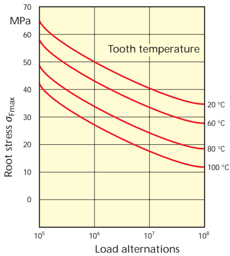
Diagram 9: Root strength of teeth \sigma_{Fmax} für POM
